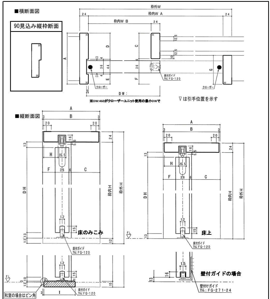
■ 横断面図・縦断面図
