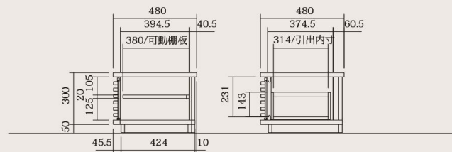
<側面図 / 共通>
