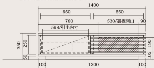
<正面図>
